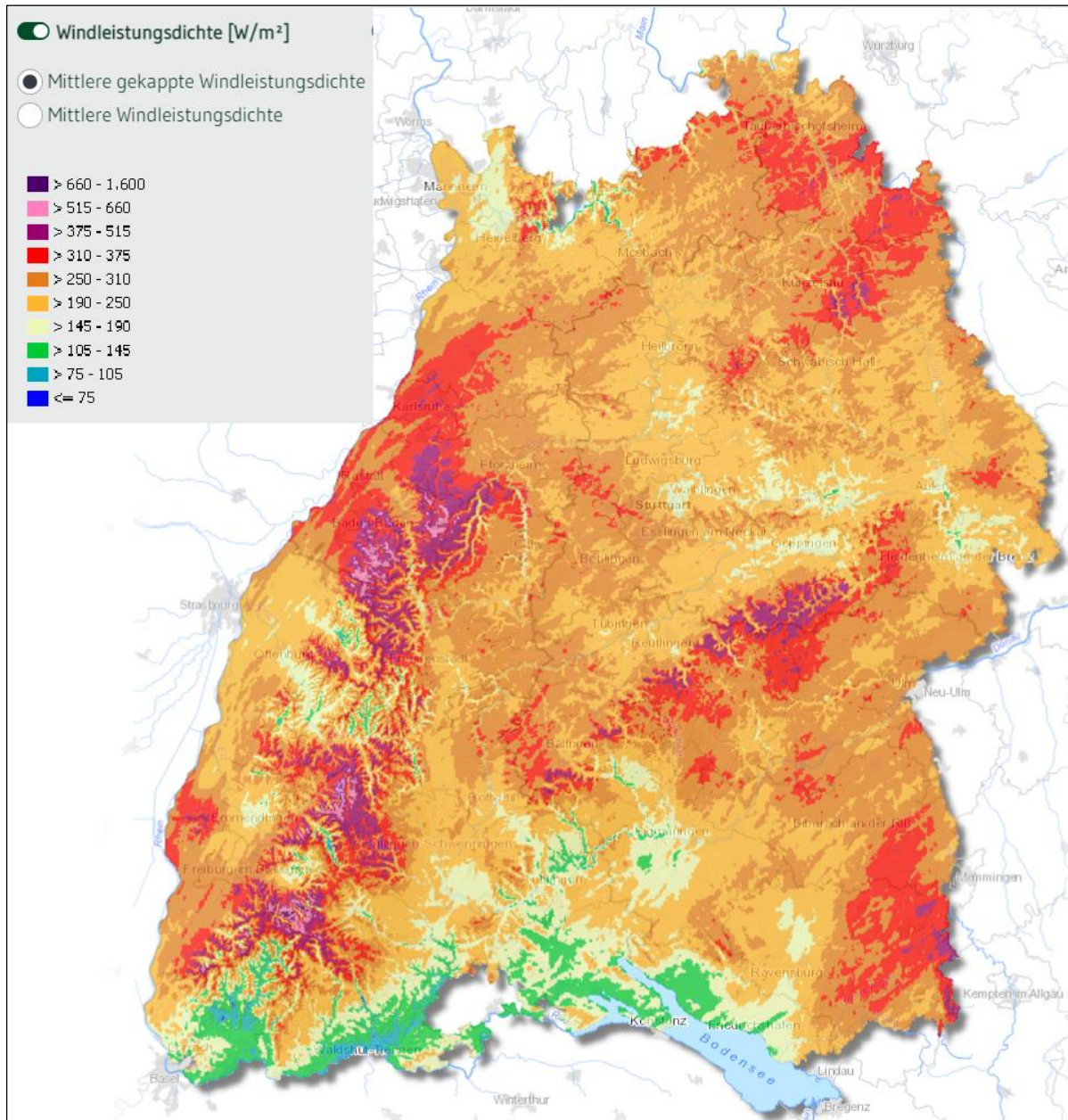
Bild 49: Gekappte Windleistungsdichte in Baden-Württemberg in 200 m Höhe 42
