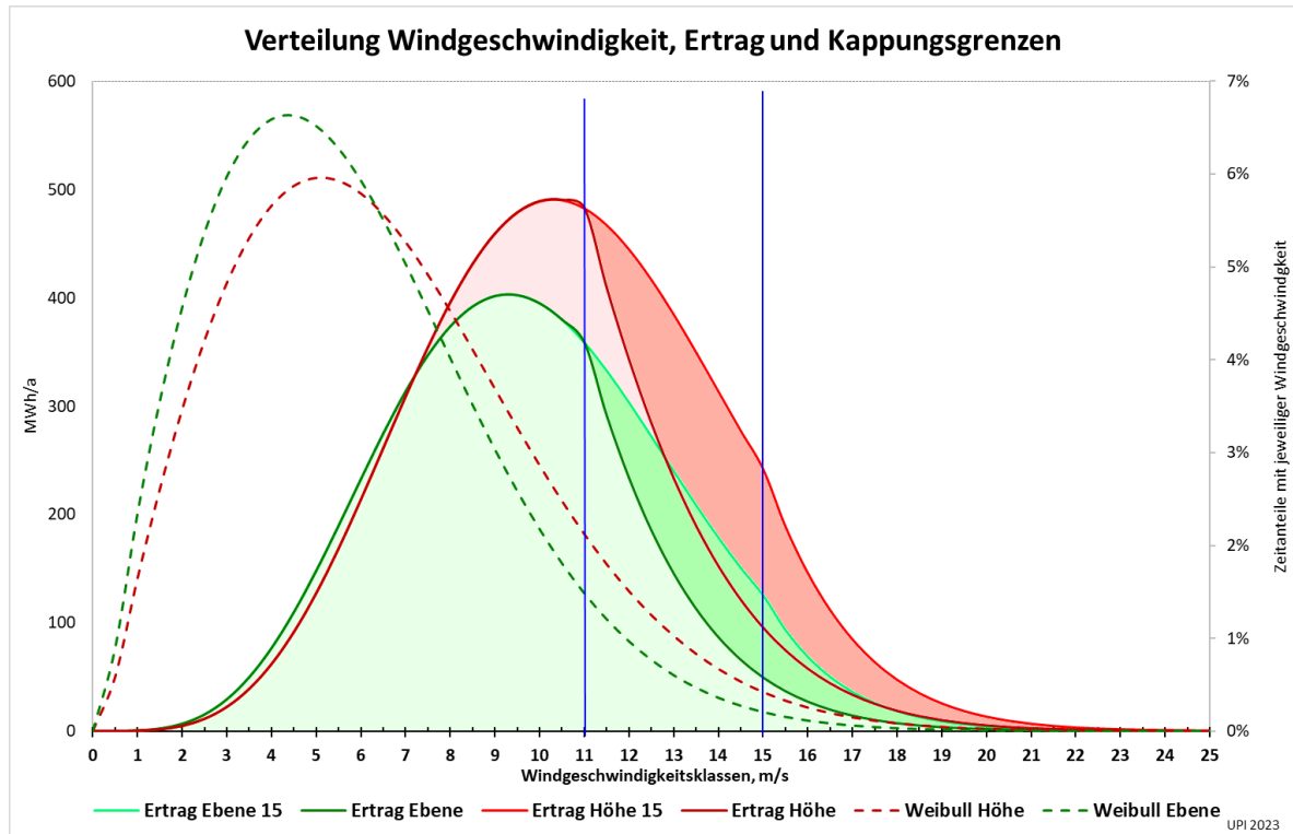
Bild 20: Einfluss der Kappungsgrenze auf den Ertrag bei Standorten in der Ebene und auf Höhen
