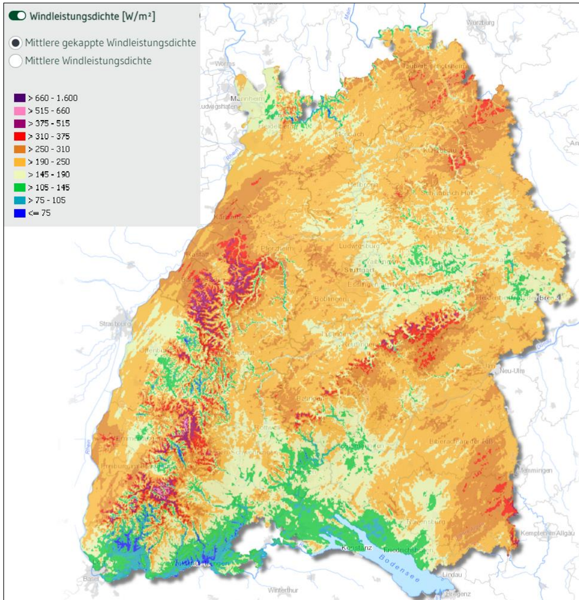
Bild 48: Gekappte Windleistungsdichte in Baden-Württemberg in 160 m Höhe 42
