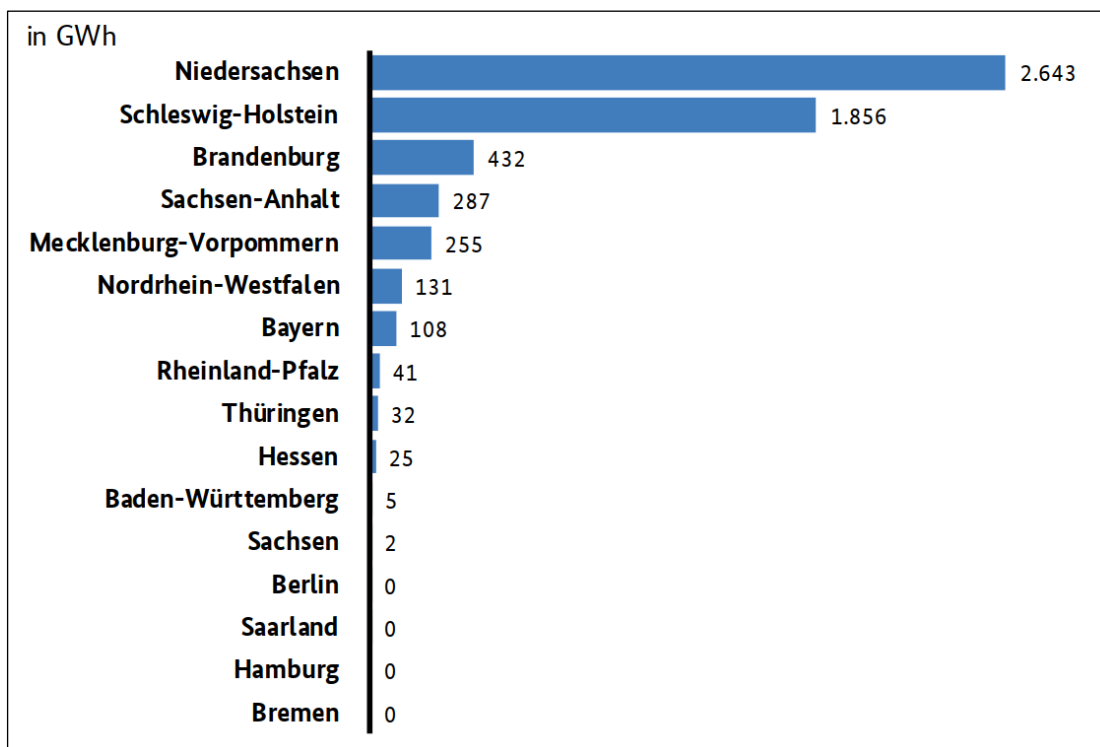
Bild 45: Regionale Verteilung der Ausfallarbeit im Jahr 2021 79
