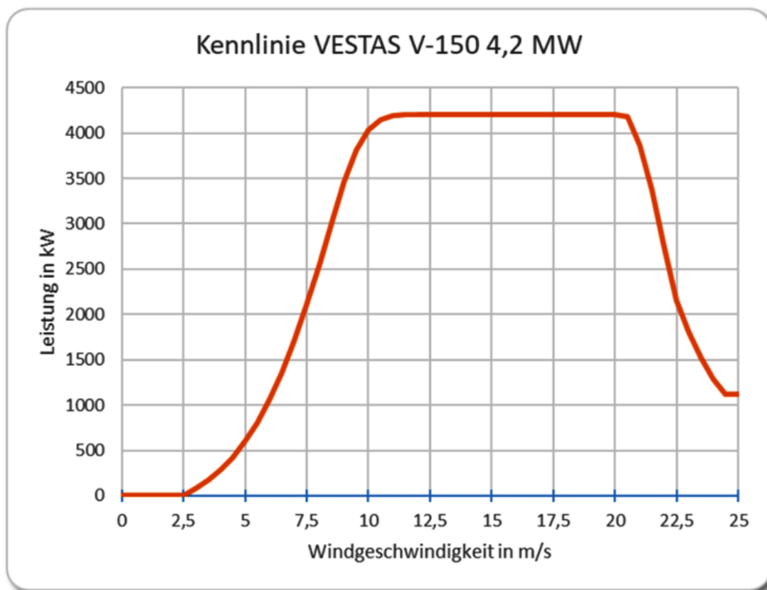
Bild 19: Leistungskennlinie eines Windkraftwerks (Vestas V-150 4,2 MW p ) bei Standardluftdichte, aus 42
