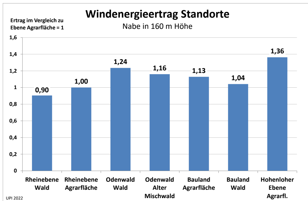
Bild 22: Vergleich des Ertrags von Windkraftwerken im Odenwald und in der Ebene
