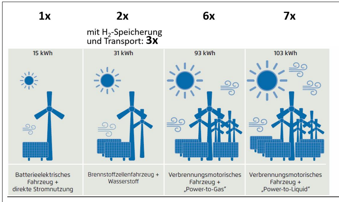
Bild 40: Bedarf regenerativen Stroms für verschiedene Antriebsarten 62
