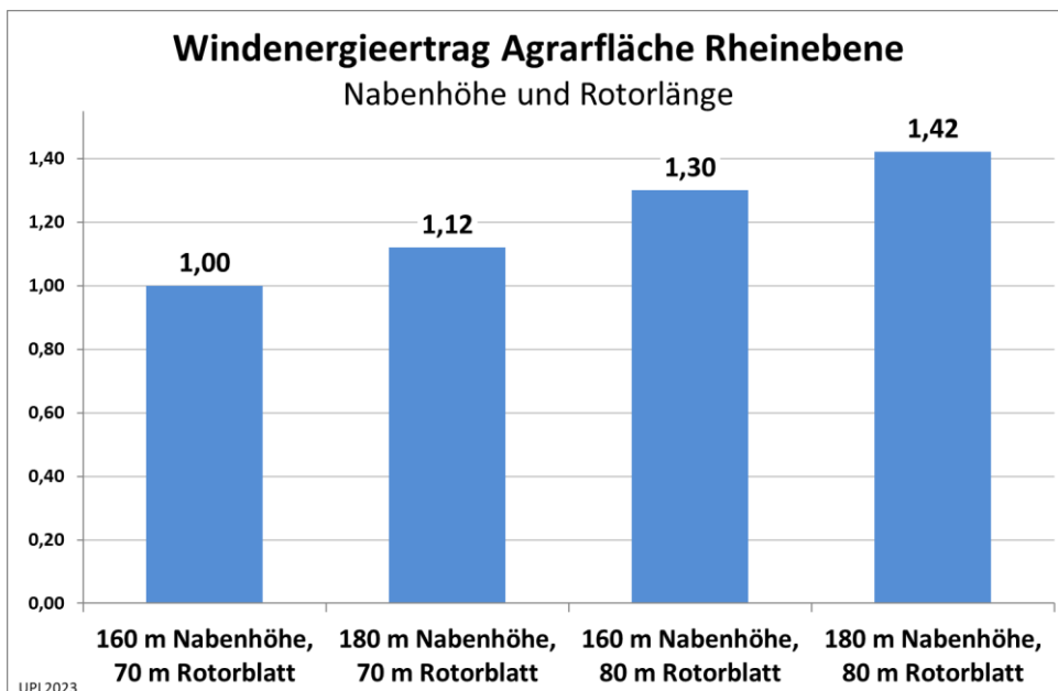
Bild 24: Einfluss von Nabenhöhe und Rotorblattlänge auf den Stromertrag von Windkraftwerken in der Ebene
