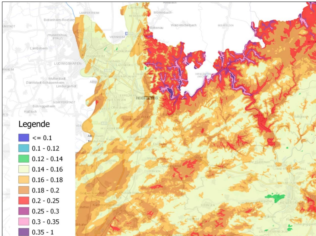
Bild 21: Mittlere meteorologische Umgebungsturbulenzintensität in 160 m Höhe 44
