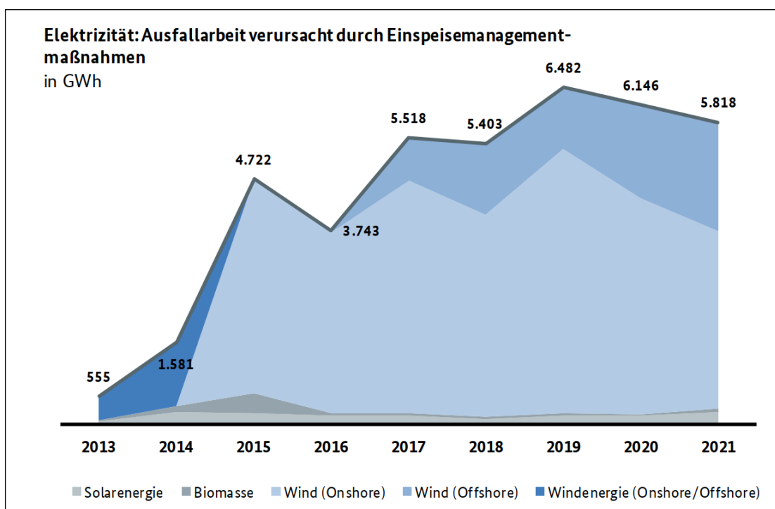
Bild 44: Ausfallarbeit verursacht durch Einspeisemanagementmaßnahmen 79
