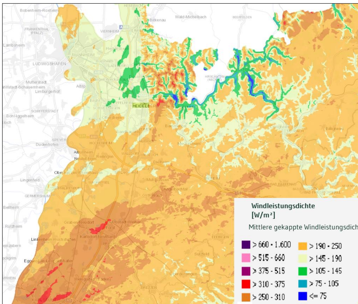
Bild 18: Ab 15 m/s gekappte Windleistungsdichte (W/m 2 ) 160 m über Grund 42
