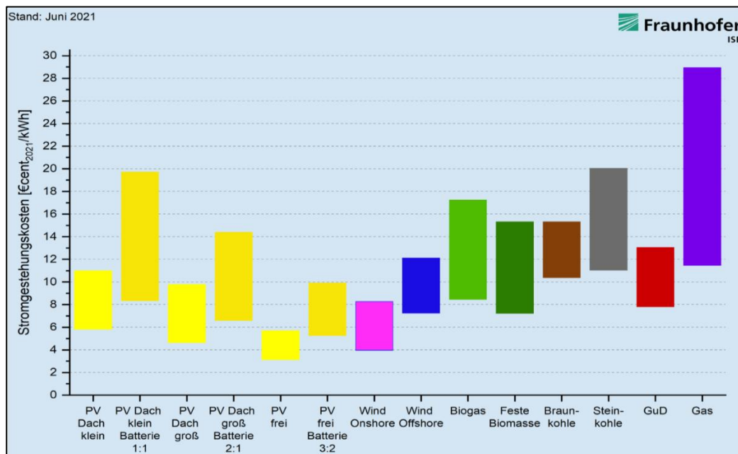
Bild 25: Stromgestehungskosten für erneuerbare Energien und konventionelle Kraftwerke an Standorten in Deutschland im Jahr 2021 50
