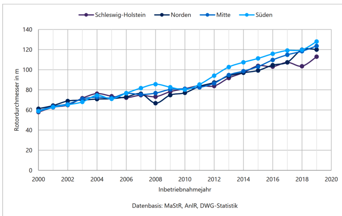
Bild 23: Mittlerer Rotordurchmesser je Inbetriebnahmejahr, aus 49 , inzwischen gibt es Schwachwindanlagen mit 160 m Rotordurchmesser
